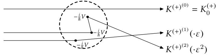
Obrázek 12: Možné dráhy částice odpovídající poruchovým členům 0., 1. a 2. řádu při průchodu interakční oblastí
