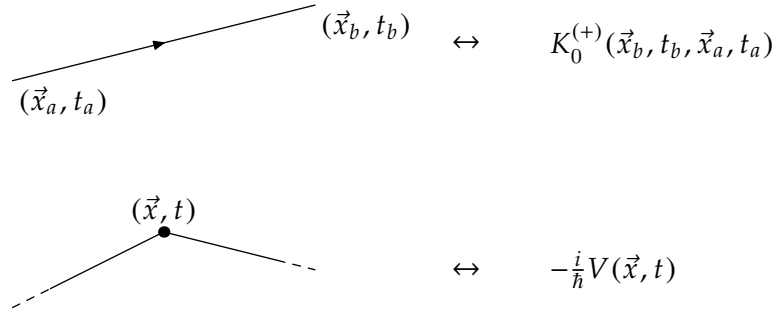
Obrázek 10: Úsečka a vrchol ve Feynmanově diagramu
