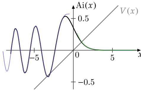
Obrázek 3: Graf Airyho funkce Ai(x) a jejích aproximací pro kladná a záporná x . Slabší čarou potenciálová funkce (v nesouvisejících jednotkách; voleno E = 0 ), již by takové řešení odpovídalo.
